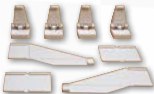
Leitplankenhalterungen 16 x, Endstücke 4 x, Verbindungsstücke 2 x Guard rail supports 16 x, end pieces 4 x, guard rail connecting pieces 2 x
